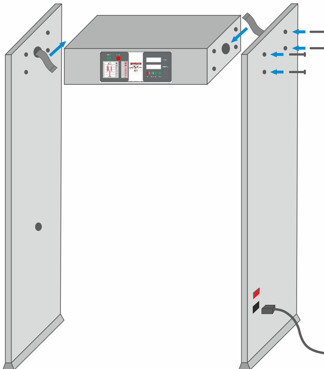
Рисунок 3. Сборка металлодетектора.
