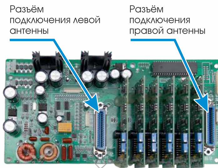
Рисунок 4. Материнская плата.
