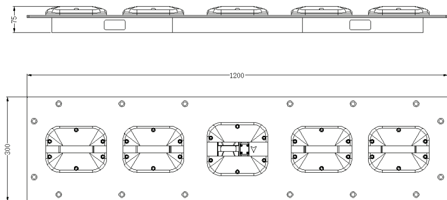
Чертеж
