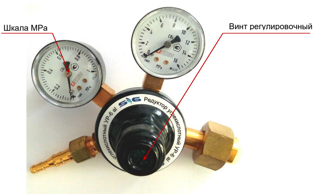
Рисунок 4 – Редуктор
