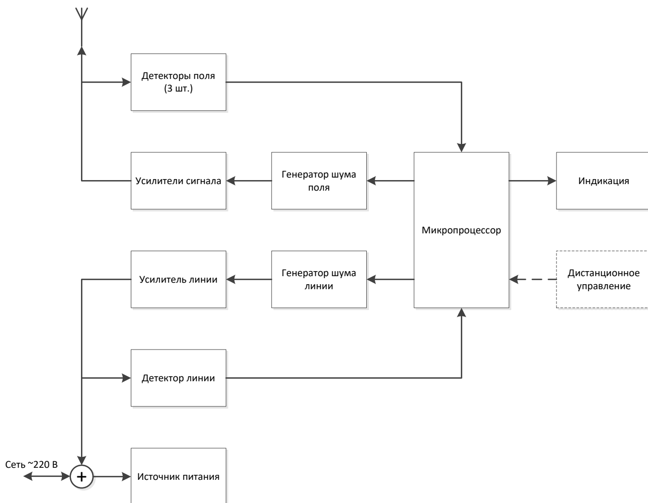
Рисунок 1 – Функциональная схема
