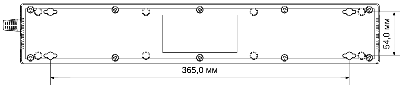
Рисунок 2 – Задняя панель Изделия
