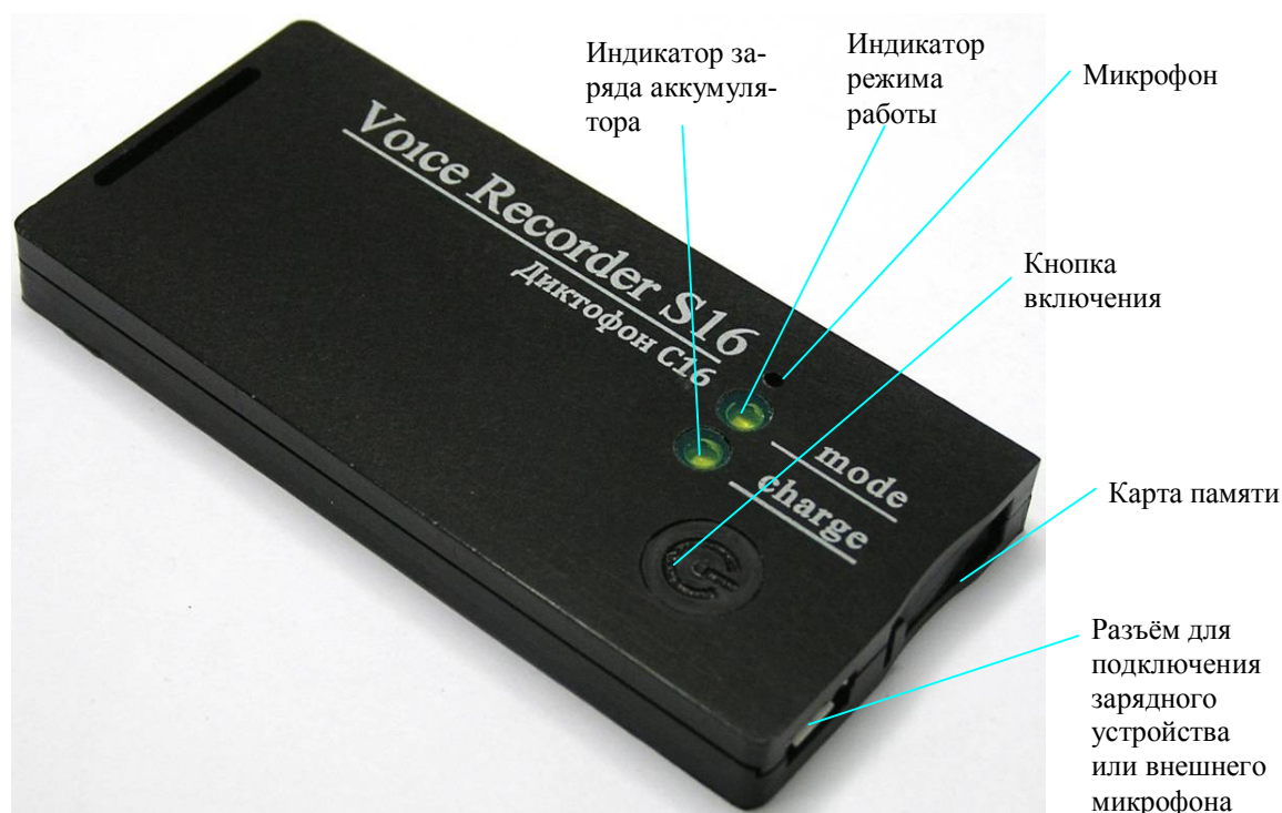
Рис. 2. Внешний вид диктофона «СОРОКА-16».
