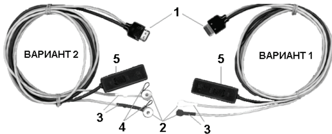
Рисунок 2 – Микрофонная гарнитура
